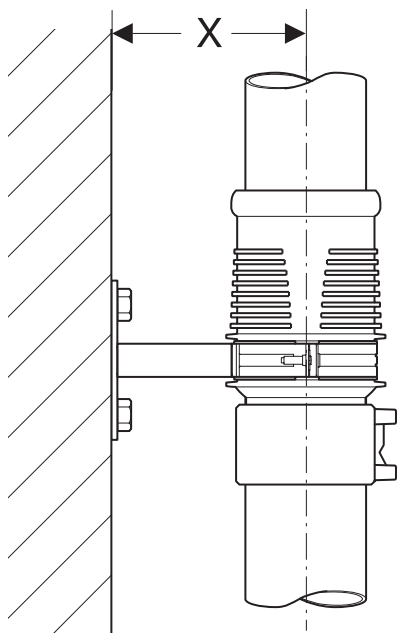
Abbildung 2: Vertikale Fixpunktbefestigung mit schallgedämmter Geberit Silent-db20 Rohrschelle auf der Geberit Silent-db20 Langmuffe.
